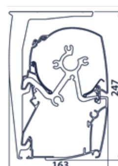
Plafondbevestiging
